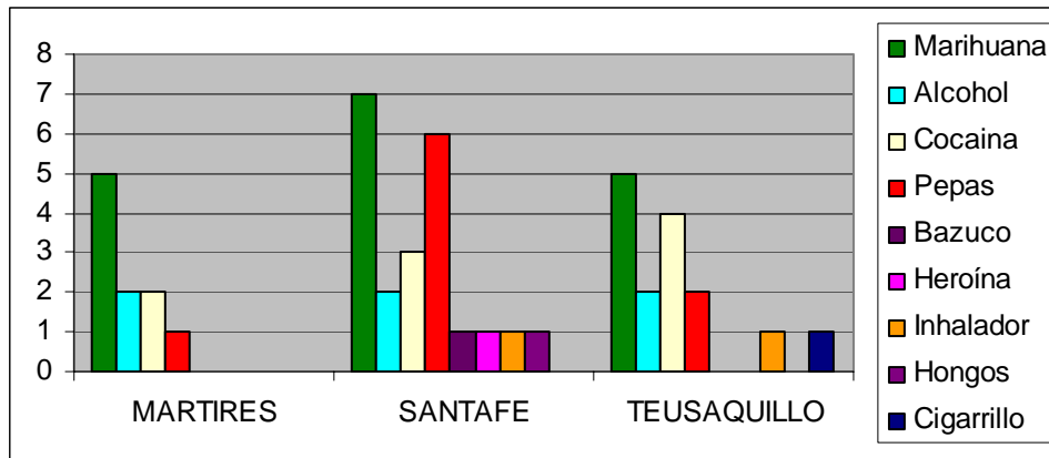
GRAFICA Nº 2 Consumo de Sustancias Psicoactivas
